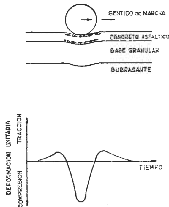
FIG. 2 PERFIL DE DEFORMACIÓN EN LA SUPERFICIE DE UN PAVIMENTO SOMETIDO A LA ACCIÓN DE UNA RUEDA SIMPLE EN MOVIMIENTO
