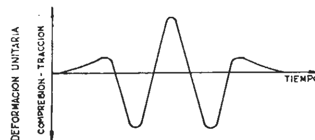
Fig. 3: PERFIL DE DEFORMACION EN UN PAVIMENTO FLEXIBLE SOMETIDO A LA ACCION DE UN MOVIL TIPO TANDEN
